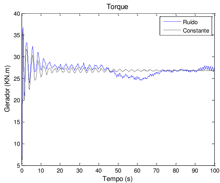
Figura 38 - Torque do Gerador (KN.m)
