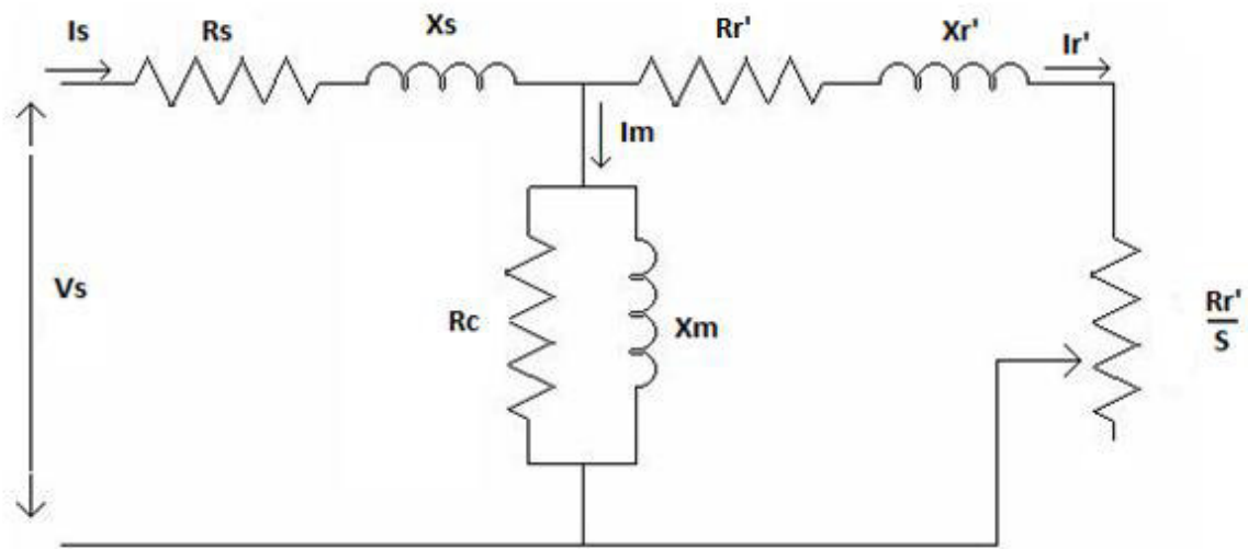
Figura 31 - Circuito Equivalente da Máquina de Indução [16]
