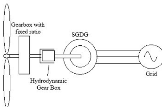
Figura 17 - Gerador Síncrono com multiplicação da caixa dinâmica [7]
