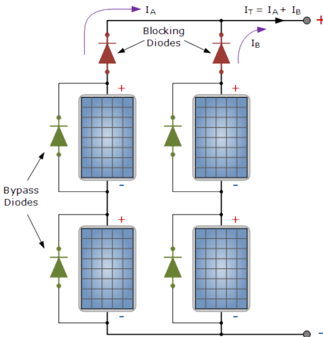
Figura 12 - Esquemático de um diodo de um sistema com diodos de by-pass para proteção. (EnergiaTecSolar, 2015)
