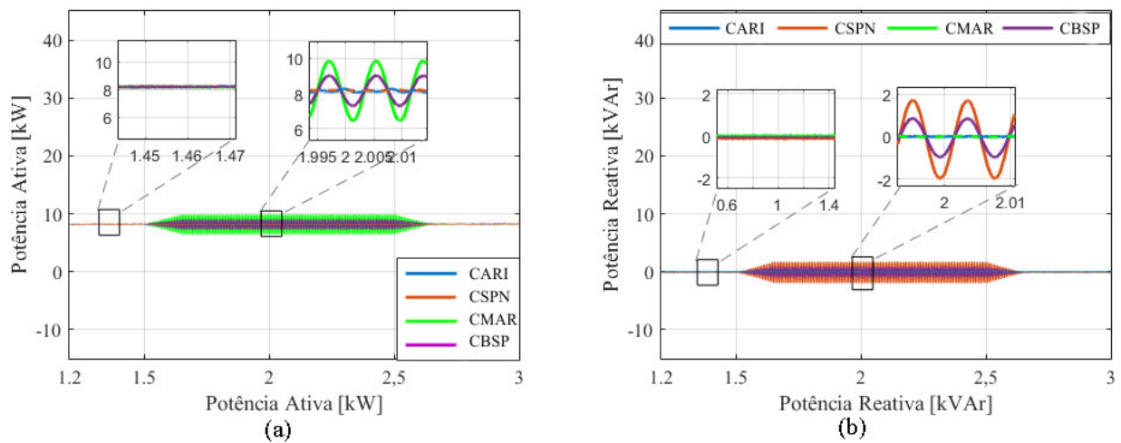
Figura 6 – Potências ativa (a) e reativa (b) injetadas na rede para as quatro estratégias.
